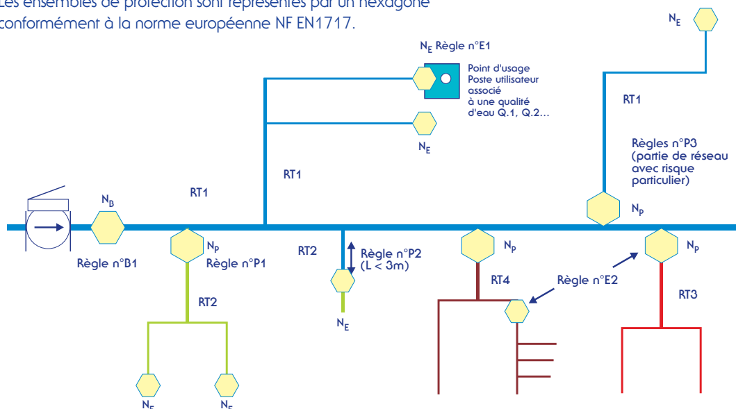
Schéma 3 : Exemple de structure d'un réseau type
