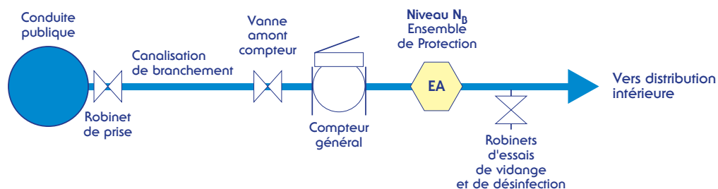
Schéma 1 : Exemple de configuration d'un branchement d'eau d'alimentation d'une distribution intérieure, raccordé à une conduite publique
