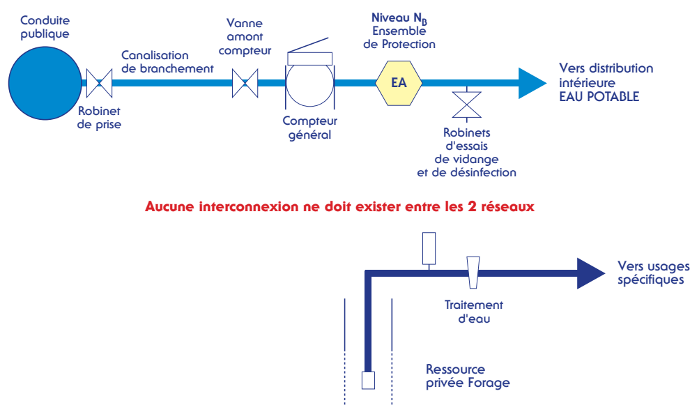
Schéma 2 : Principe de séparation des réseaux d'eau
